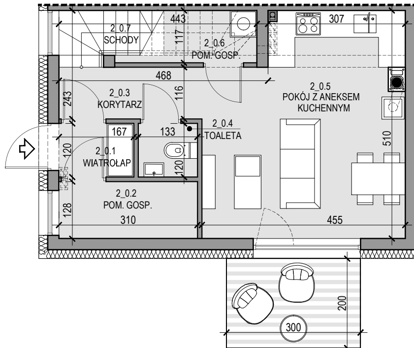
RZUT PARTERU
