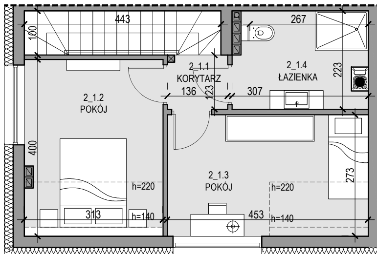
RZUT PIĘTRA
