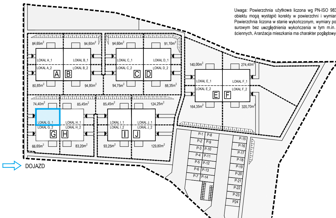
RZUT PIĘTRA
