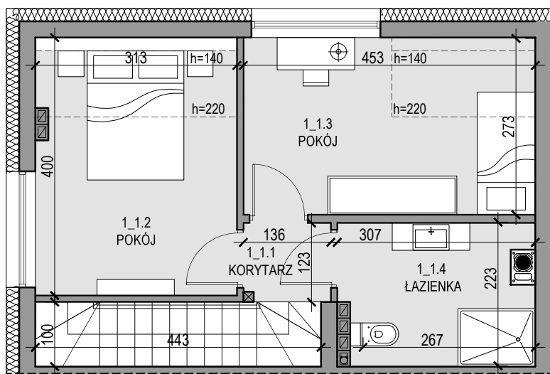
RZUT PIĘTRA
