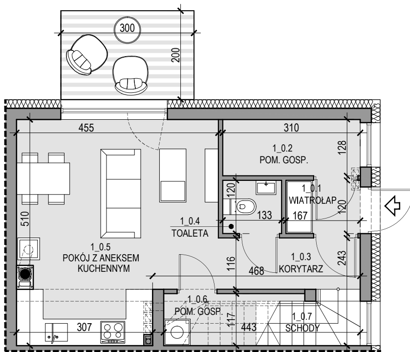
RZUT PARTERU
