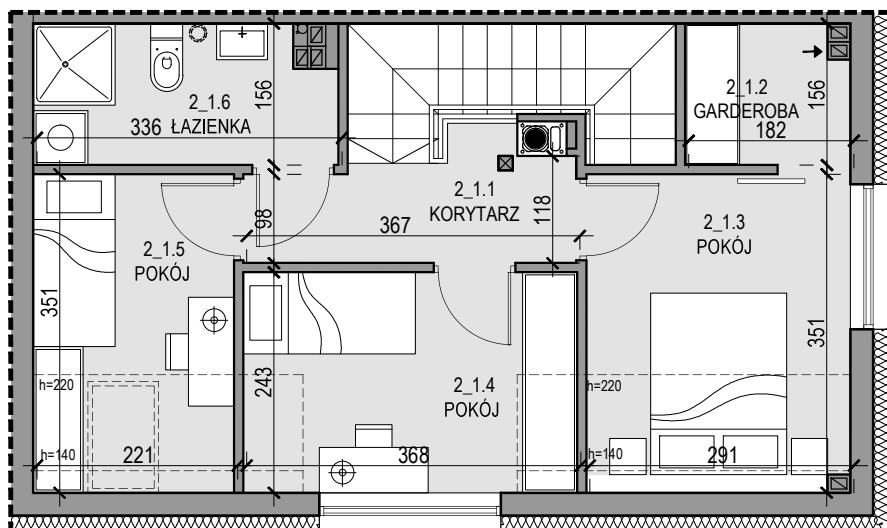
RZUT PIĘTRA
