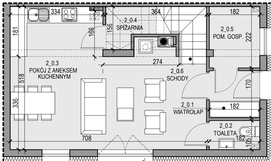
RZUT PARTERU
