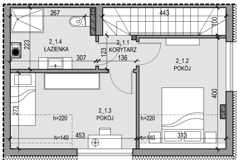
RZUT PIĘTRA
