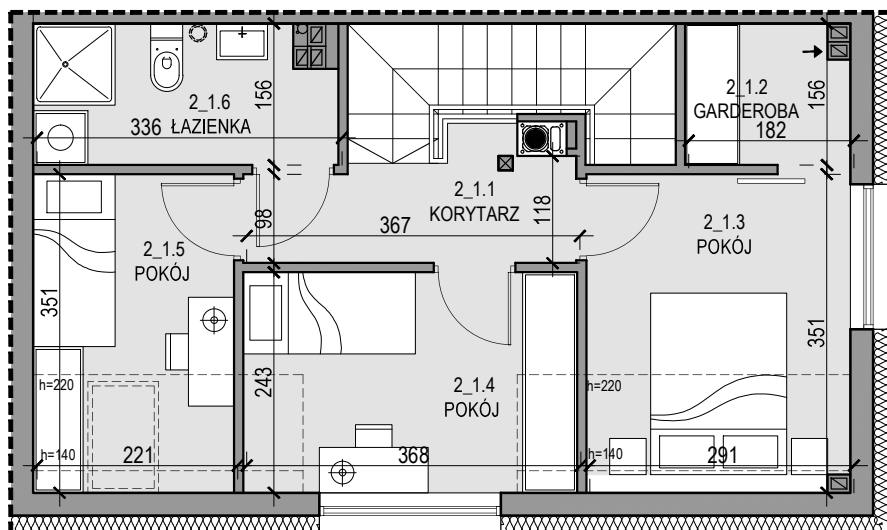
RZUT PIĘTRA
