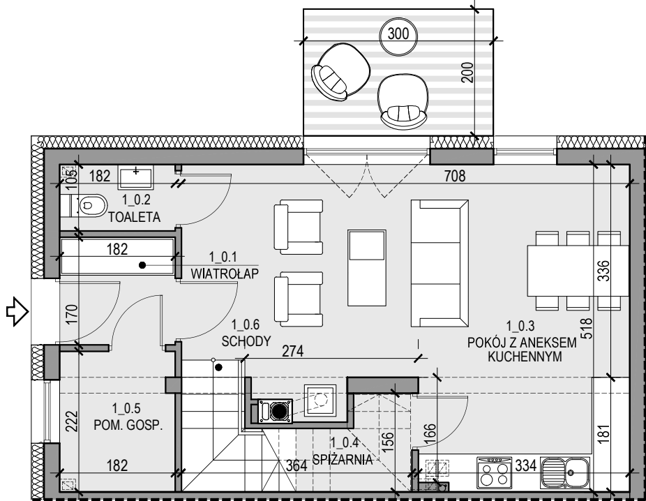
RZUT PARTERU
